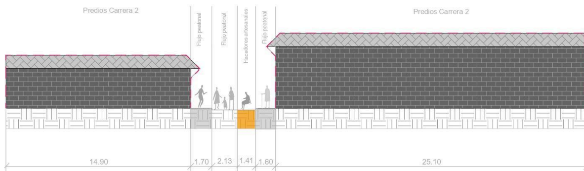
1 Perfil Vial A103 1 : 200
