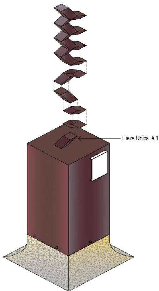
VISTA AXONOMÉTRICA EXPLOTADA ESQUEMÁTICA Sin escala
